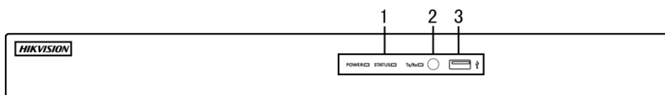
Figure 1. 3 Přední panel modelu DS-7216HGHI-SH
